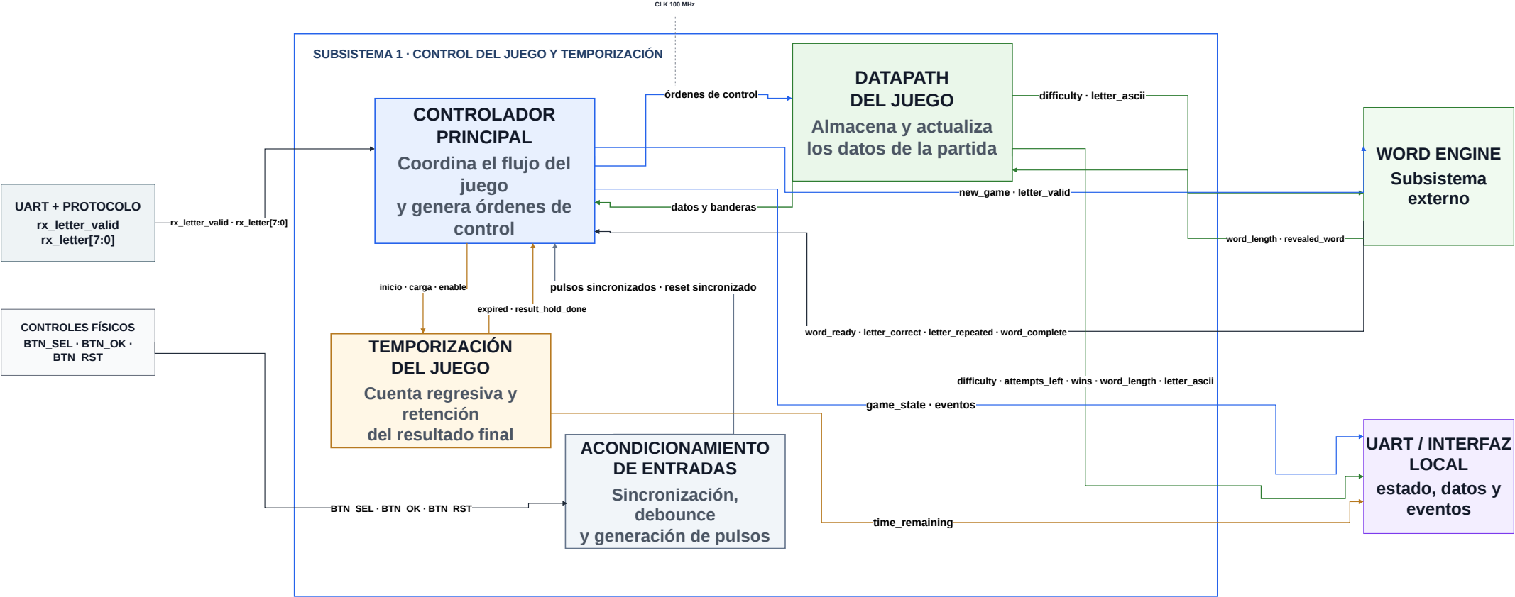
Diagrama de Segundo Nivel — Subsistema 1: Control del Juego y Temporización
